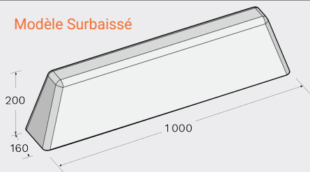
Modèle 1 m
