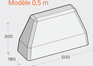
Modèle 0,5 m
