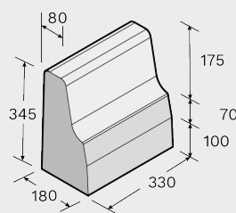
Élément droit 0,33 m
